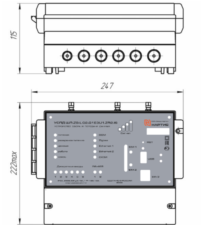
Рисунок Б.1- Габаритные и установочные размеры УСПД
