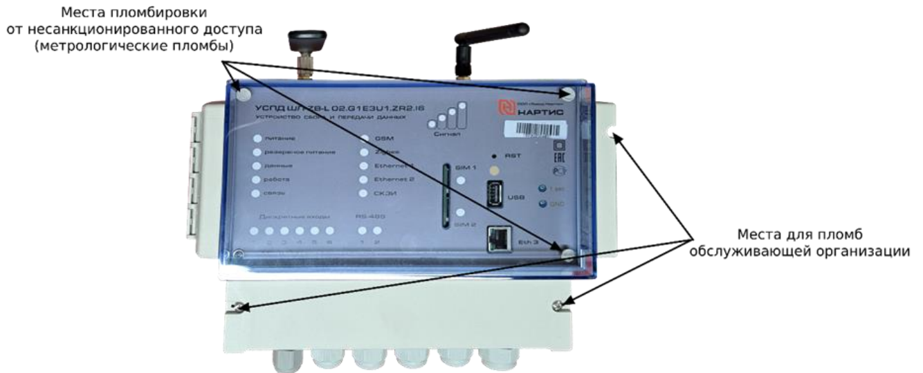
Рисунок 2 – Схема пломбировки УСПД
