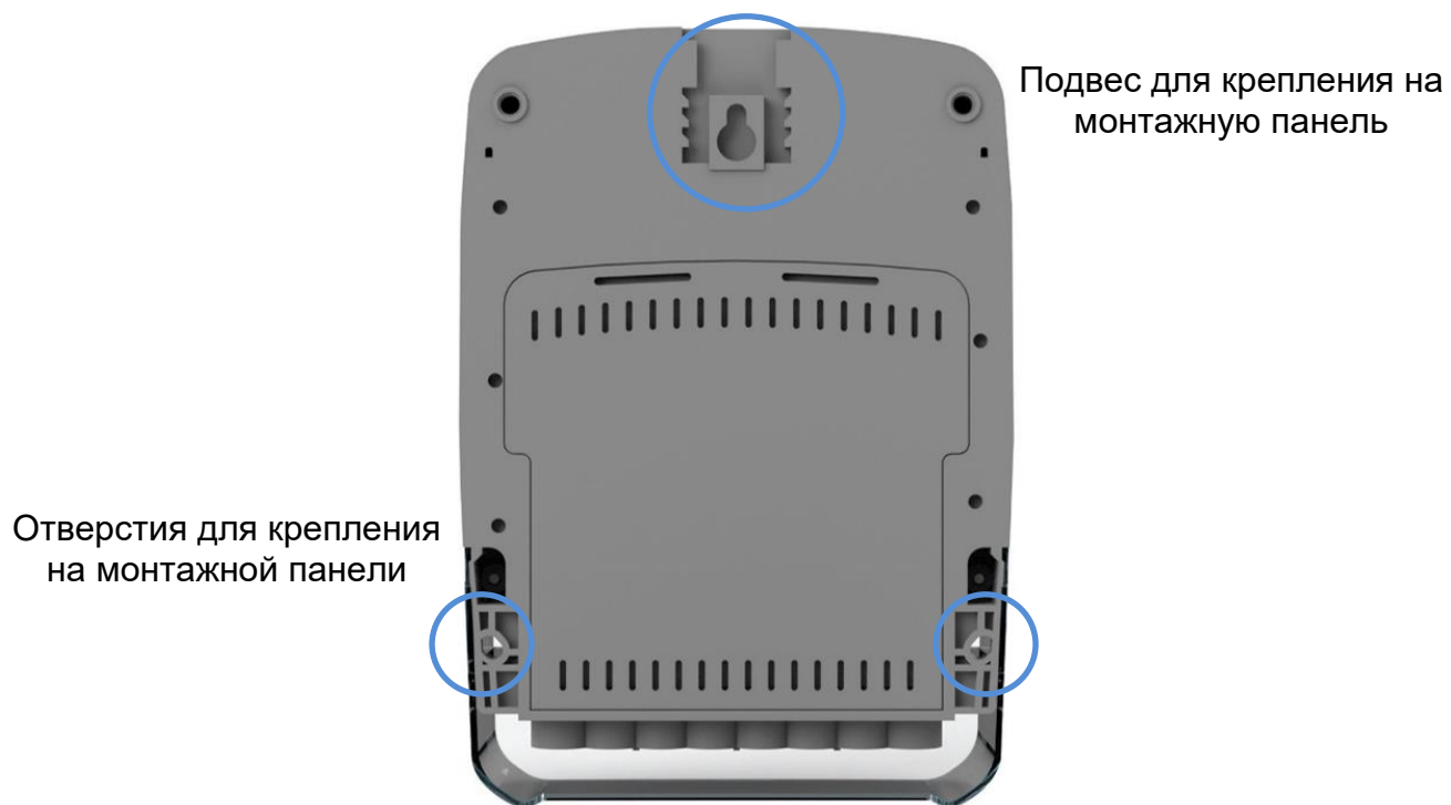
Рисунок 4 – Расположение крепежных отверстий и подвесов счетчика НАРТИС-300-W131
