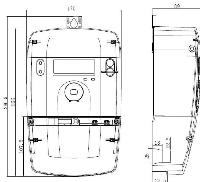
Рисунок 3 – Габаритные размеры счетчика НАРТИС-И300-W131
