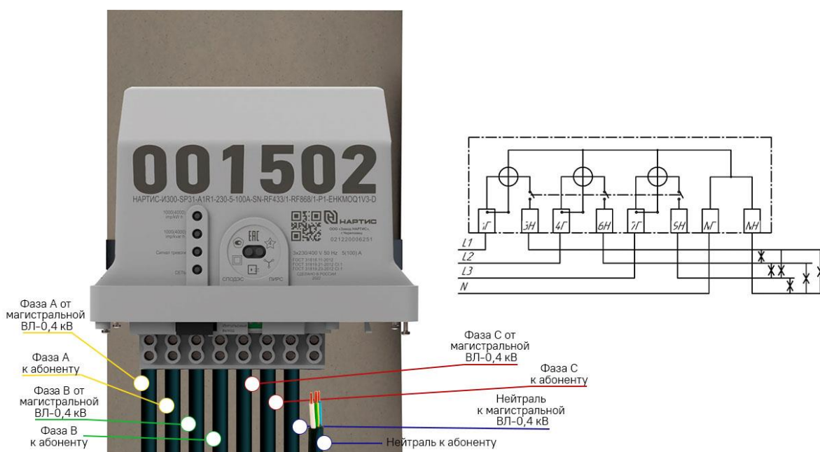
Рисунок 9 – Подключение блока измерительного счетчика НАРТИС-И300-SP31
