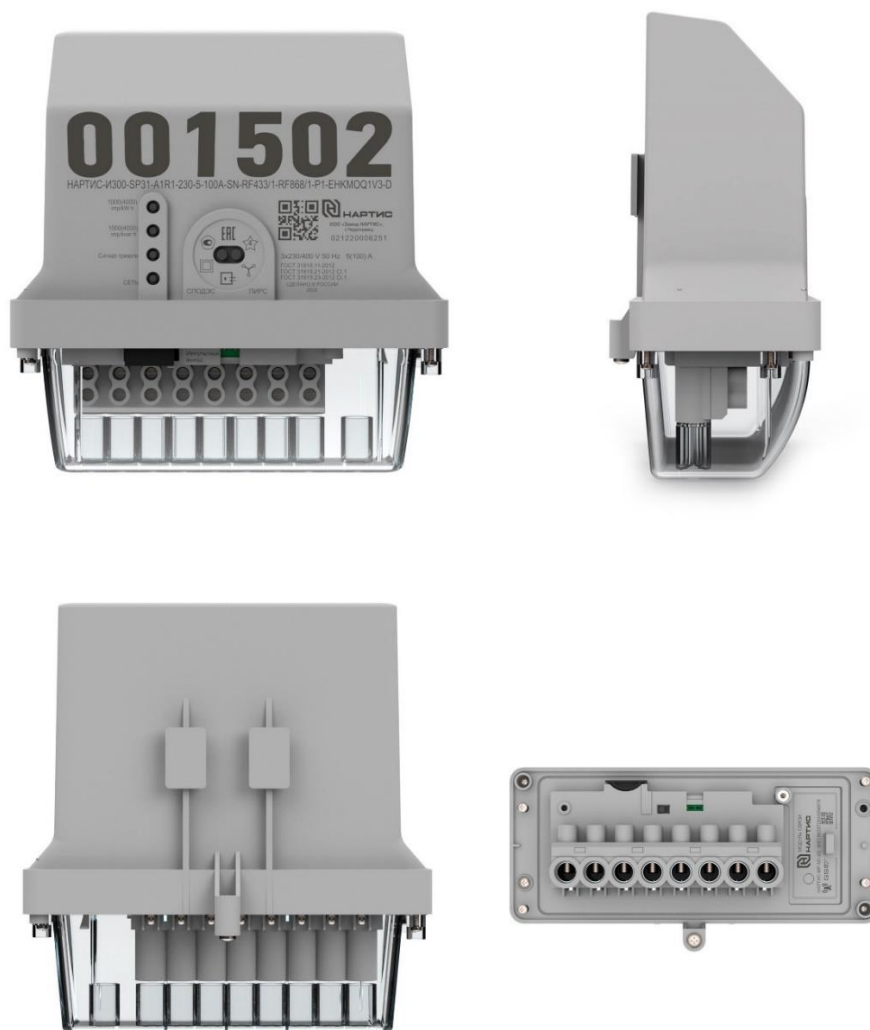
Рисунок 1 – Внешний вид счетчика НАРТИС-И300-SP31
