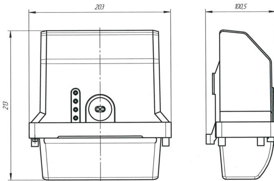
Рисунок 4 – Габаритные размеры счетчика НАРТИС-И100-SP1
